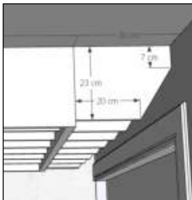
Detalhe de medidas, Armário lateral direito.
