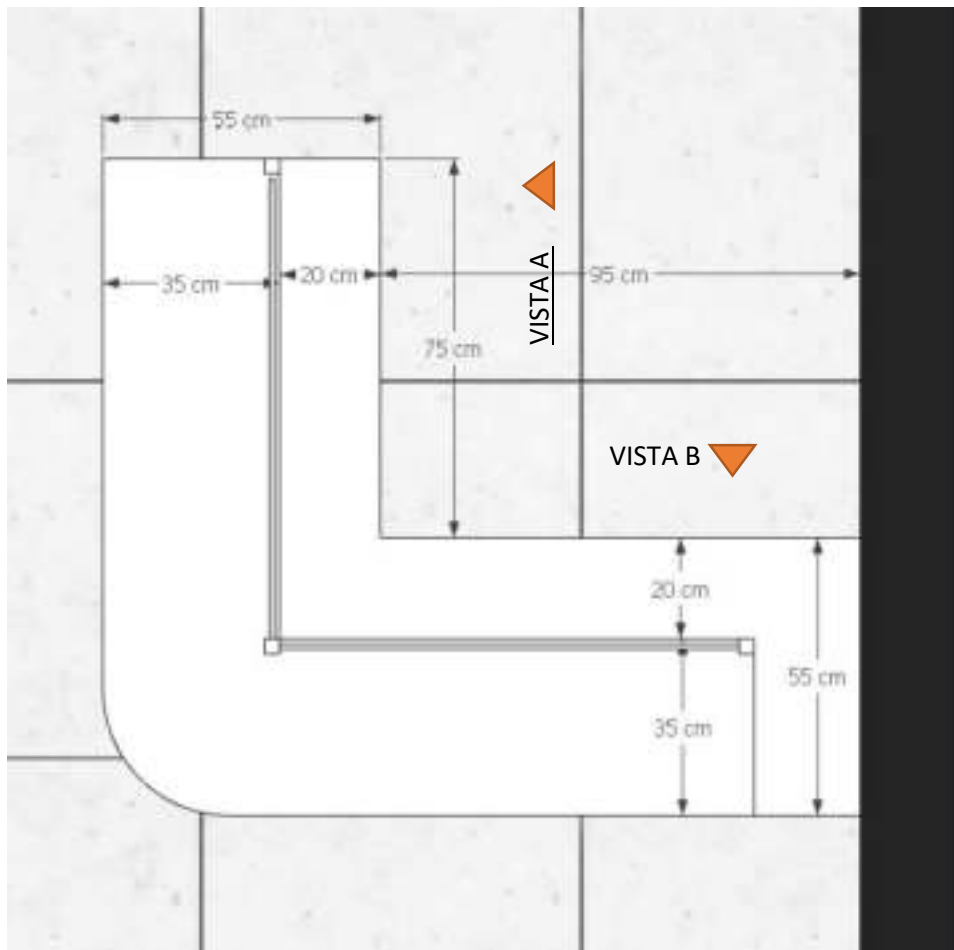
Planta baixa – Recepção
