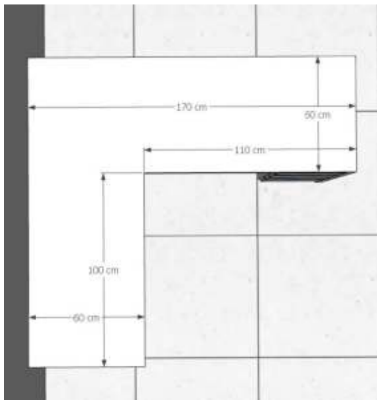
Planta Baixa do móvel Sala O2
