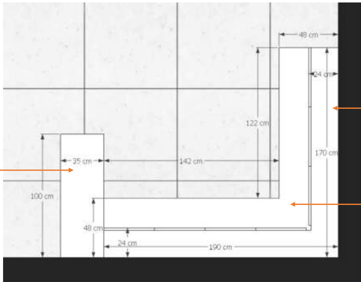
Planta Baixa Triagem
