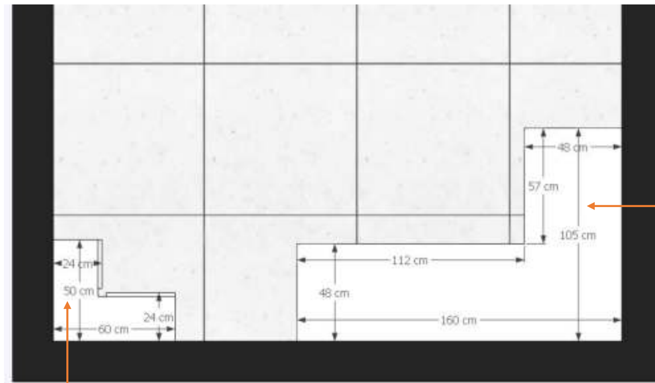
Planta Baixa do móvel Sala O3
