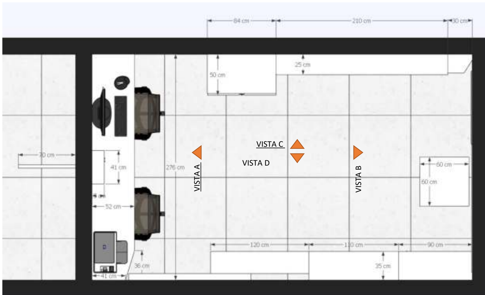
Planta baixa – Atendimento Farmácia
